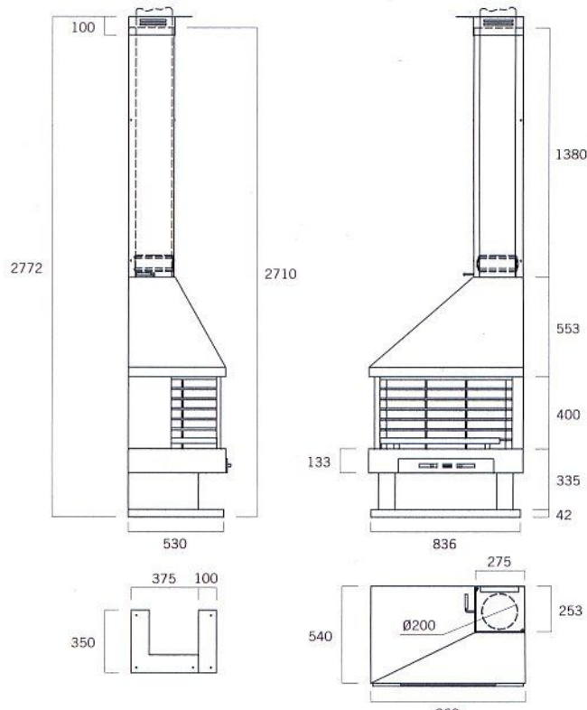
X-1205 Daril derecha/bonnes/right (según dibujo/selon schéma/as per diagram). X-1200 Daril izquierda/gouches/left
