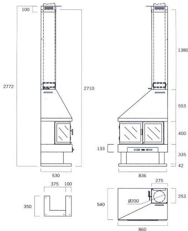
X-1206 Daril derecha con puertas/bonnes avec portes/right with doors (según dibujo/selon schéma/as per diagram).
